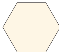
regelmäßiges Sechseck
