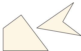
beliebige Vierecke
