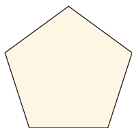
regelmäßiges Fünfeck
