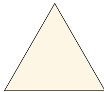
gleichseitiges Dreieck
