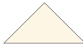
rechtwinkliges Dreieck
