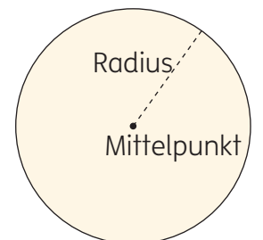
Kreis
