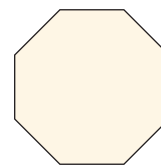
regelmäßiges Achteck
