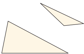
beliebige Dreiecke
