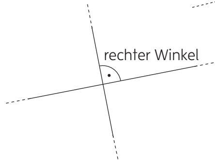
senkrechte Geraden
